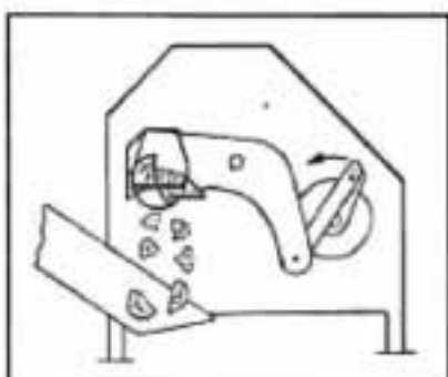
Bild 35: Arbetsprincip
